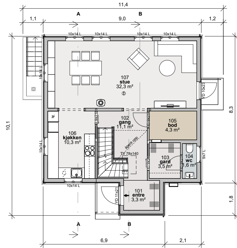
1. Etasje 1 : 100
