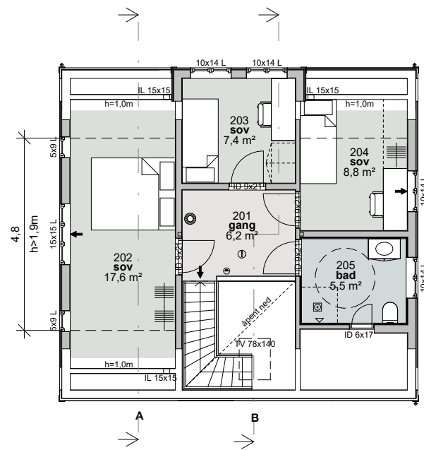
2. Etasje 1 : 100
